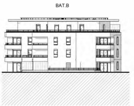
ELEVATION NORD-EST_BAT.B
